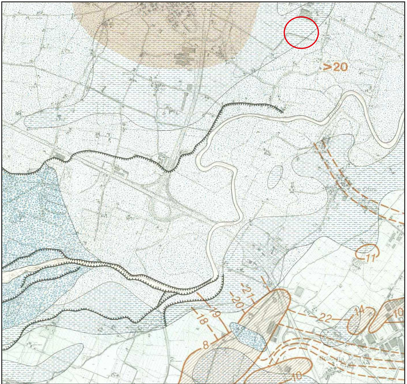
Tav. n. 5 "Carta della litologia di superficie e delle isobate del tetto del primo livello ghiaioso" Scala 1: 25000
