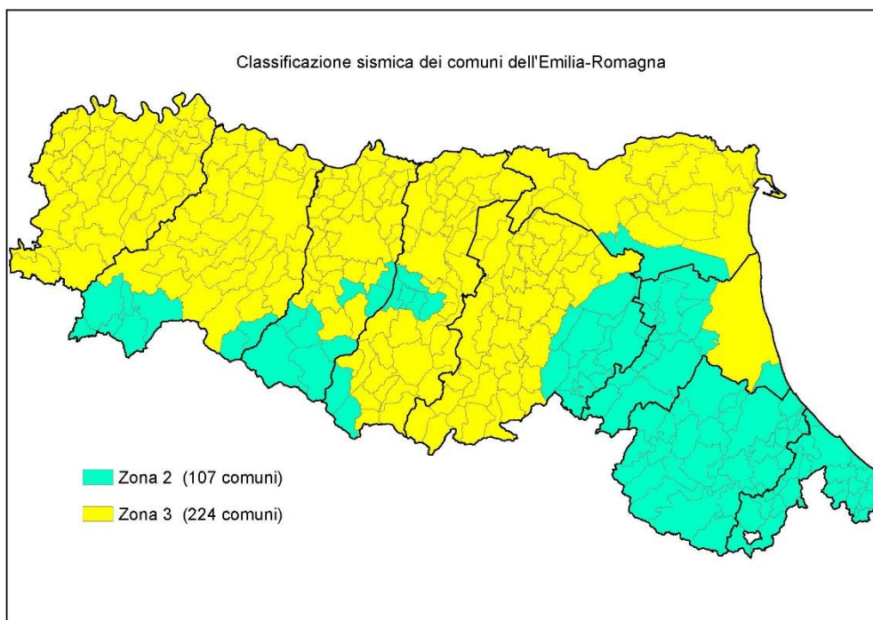
Fig. 6.1 – Classificazione sismica vigente dei comuni della regione Emilia-Romagna
