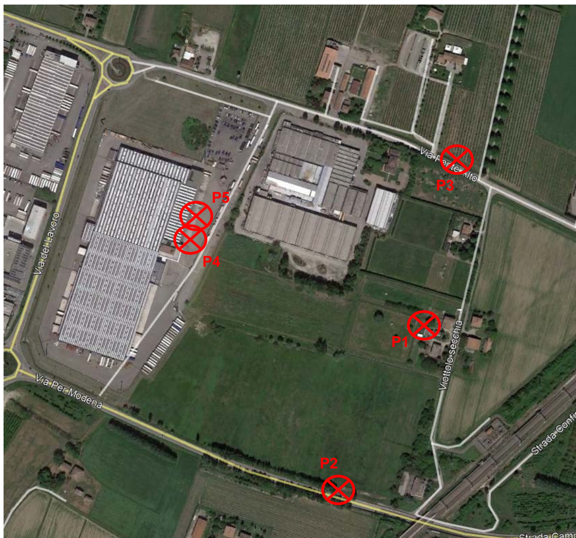
Img. 4.2 – Localizzazione delle postazioni di misura
