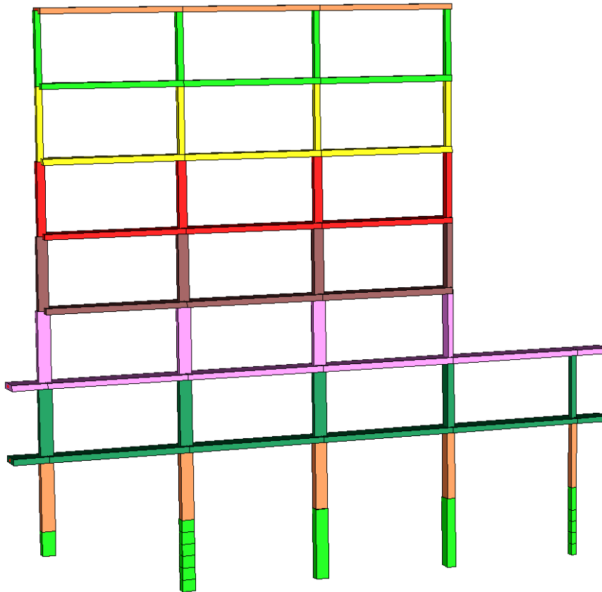
TELAIO TIPO ALL'INTERNO DEL FABBRICATO "A"
