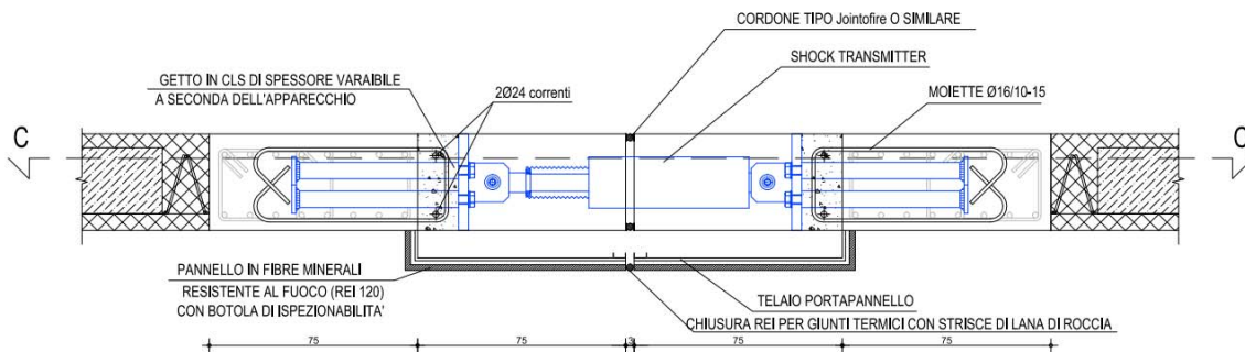
Sezione C-C
