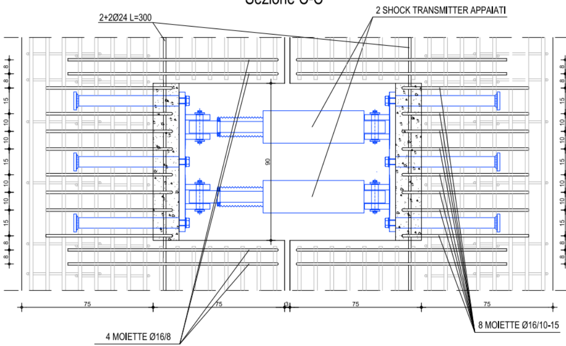
Sezione C-C
