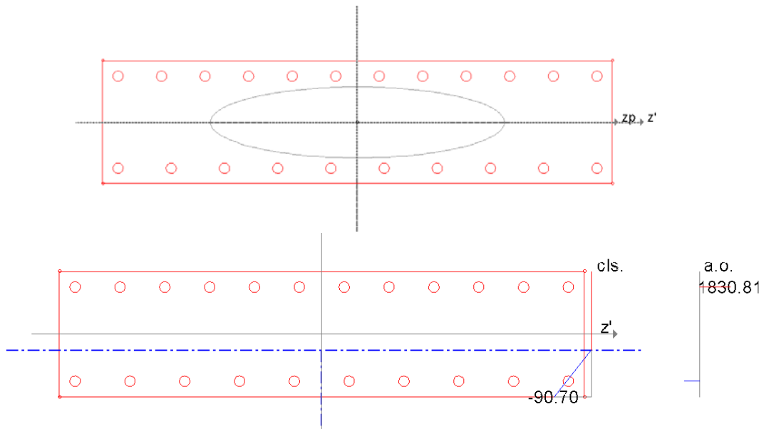
Condizione di verifica all'appoggio per massimo momento negativo
