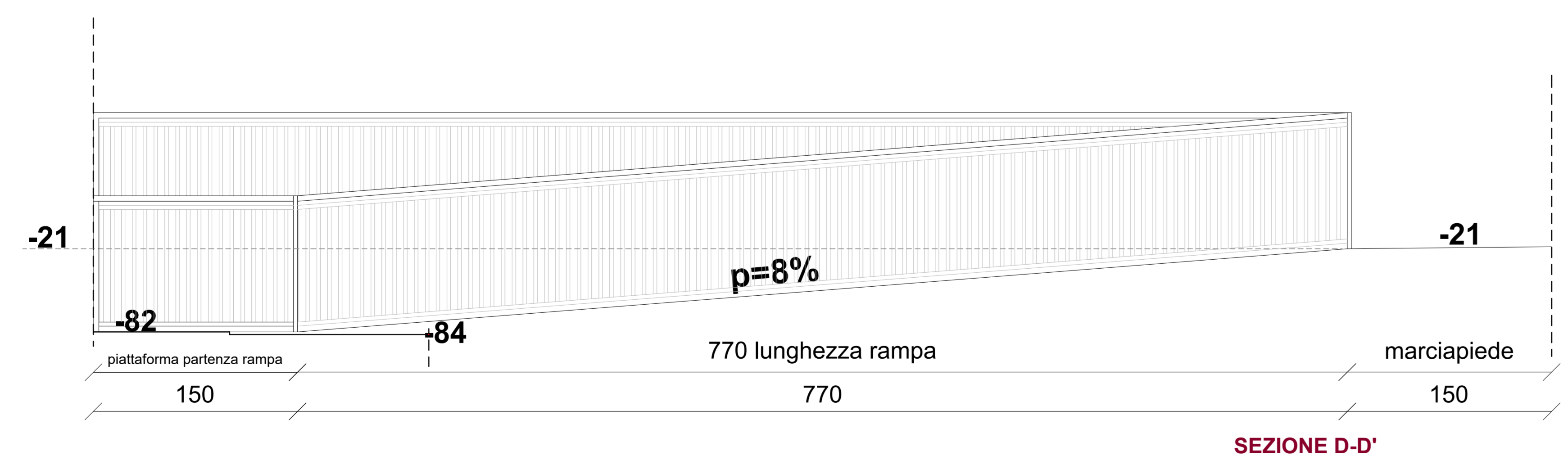
SEZIONE D-D'
